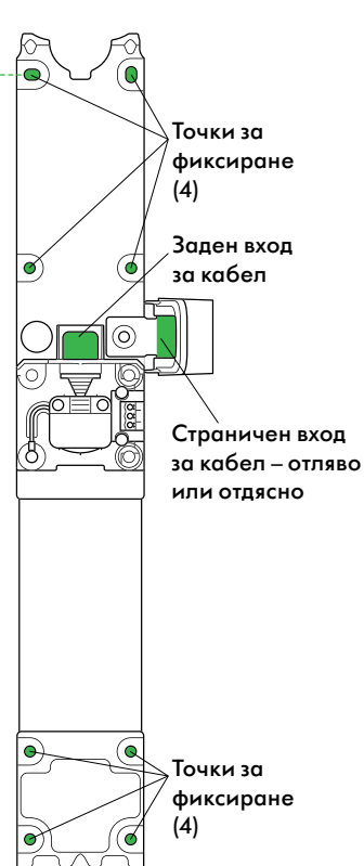
Задна планка
