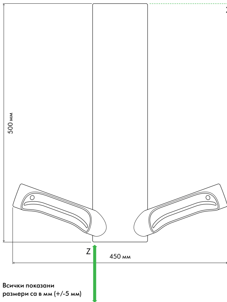
Изглед отпред
